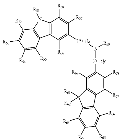
<Formula 300>
