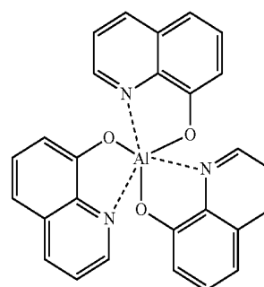
Alq
