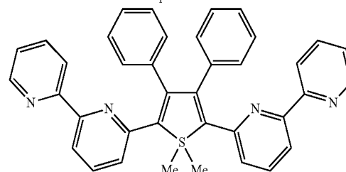
PyPySPyPy
