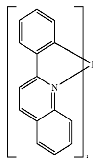
Ir(2-phq) 3
