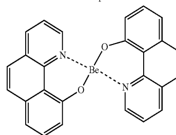
Bebq
