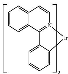
Ir(piq) 3
