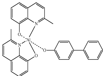
BAlq
